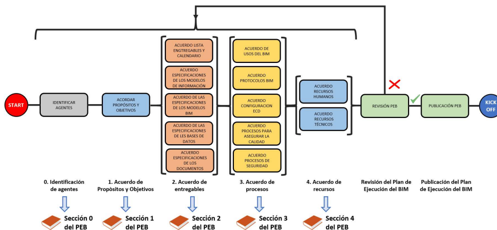
Ejemplo de Protocolo de Inicio (Este gráfico puede verse de forma ampliada en el Anejo gráfico)
